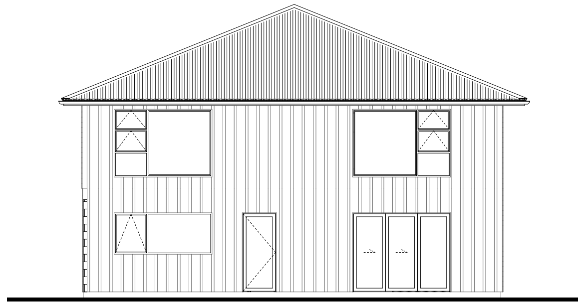
ELEVATION 1
